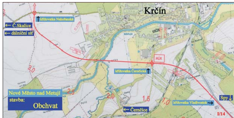
Obr.: Trasa obchvatu před Vladivostkem odbočuje ze silnice od Spů okolo bývalé cihelny přes trať a pole ke křižovatce s Černčickou ulicí, za firmou HALLA vede ke splavu na Metuji, okolo zemědělského areálu za Krčínem ke křižovatce se silnicí na Nahořany.
