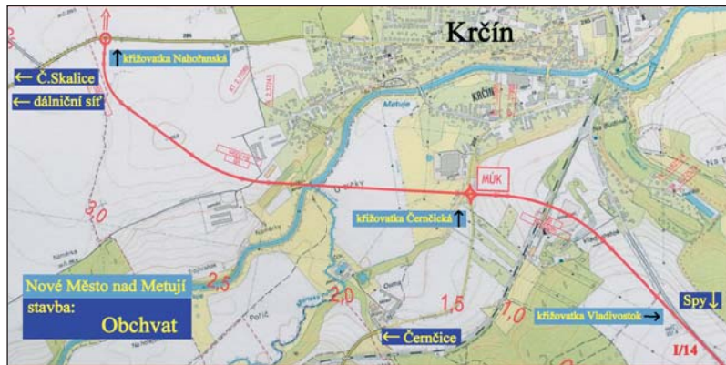
Obr.: Trasa obchvatu před Vladivostokem odbočuje ze silnice od Spů okolo bývalé cihelny přes trať a pole ke křižovatce s Černčickou ulicí, za firmou HELLA vede ke splavu na Metují, okolo zemědělského areálu za Krčínem ke křižovatce se silnicí na Nahořany.
