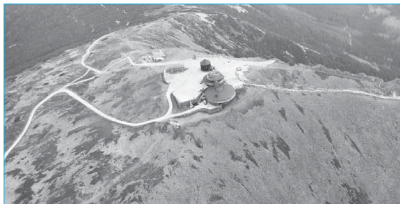
Vrcholové partie Sněžky.
